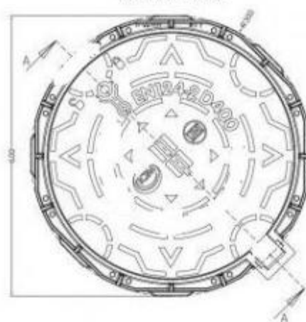
VISTA SUPERIORE
