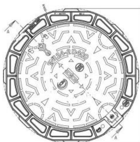
VISTA SUPERIORE
