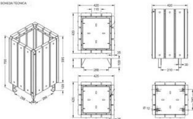
SECCION TECNICA
